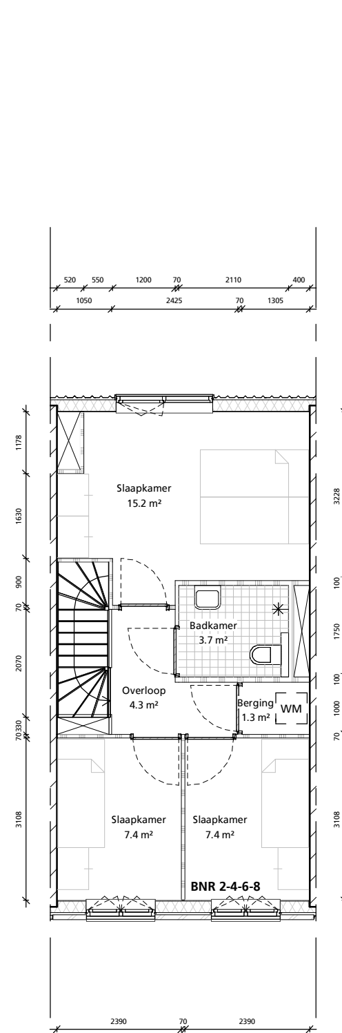
tweede verdieping
