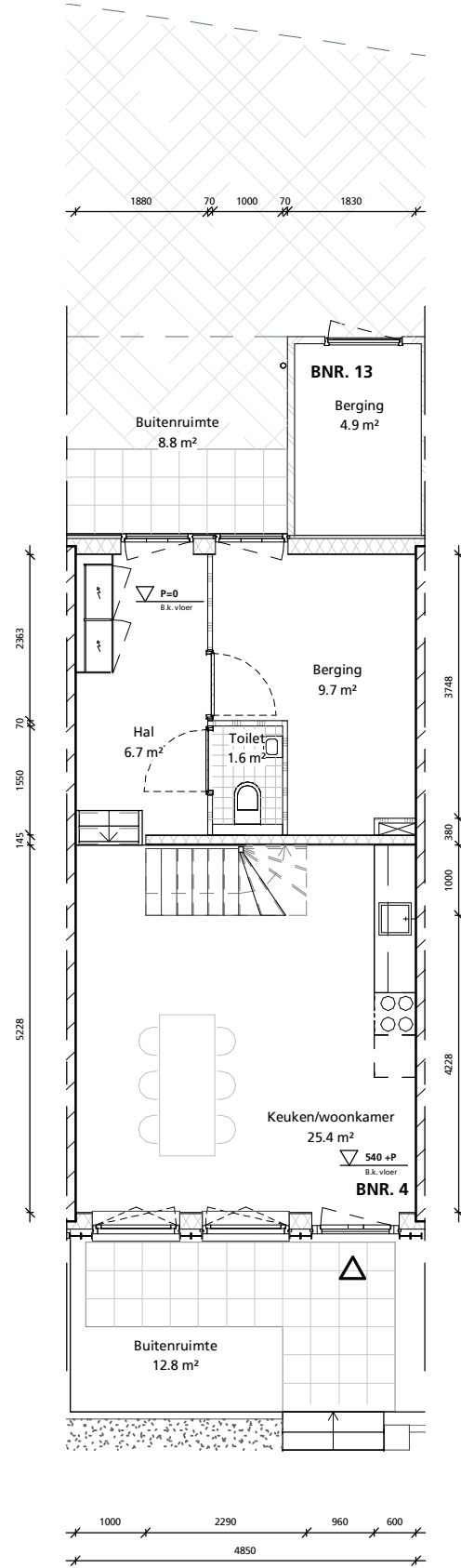
begane grond
