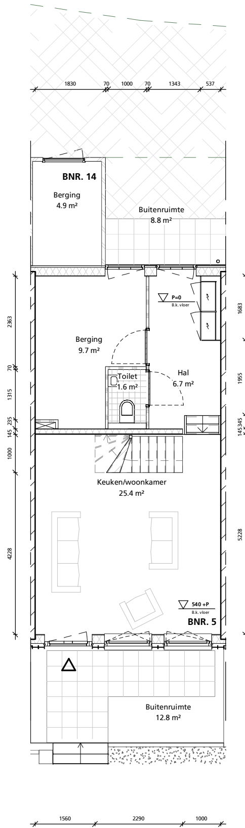
begane grond
