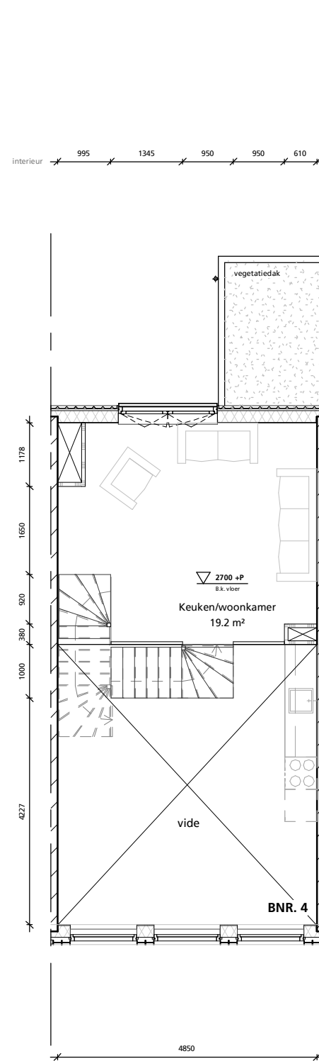
eerste verdieping
