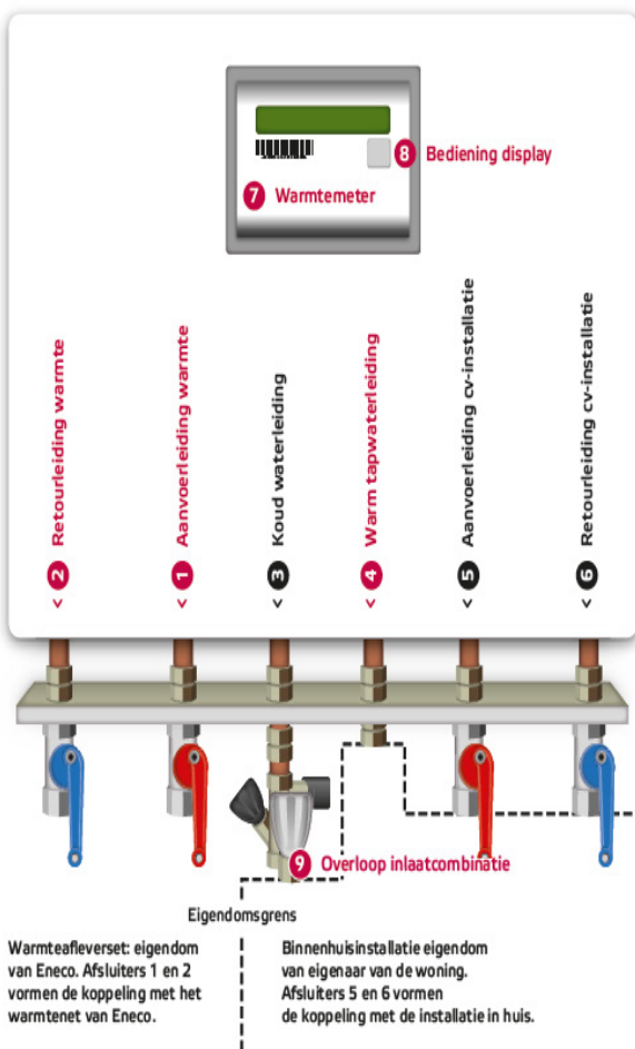
Foto 4: Warmteafleverzet met verbruiksmeter Eneco
